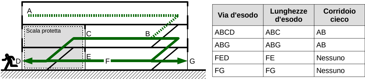
Illustrazione G.1-4: Esempi di lunghezza d'esodo e corridoio cieco, in sezione.
